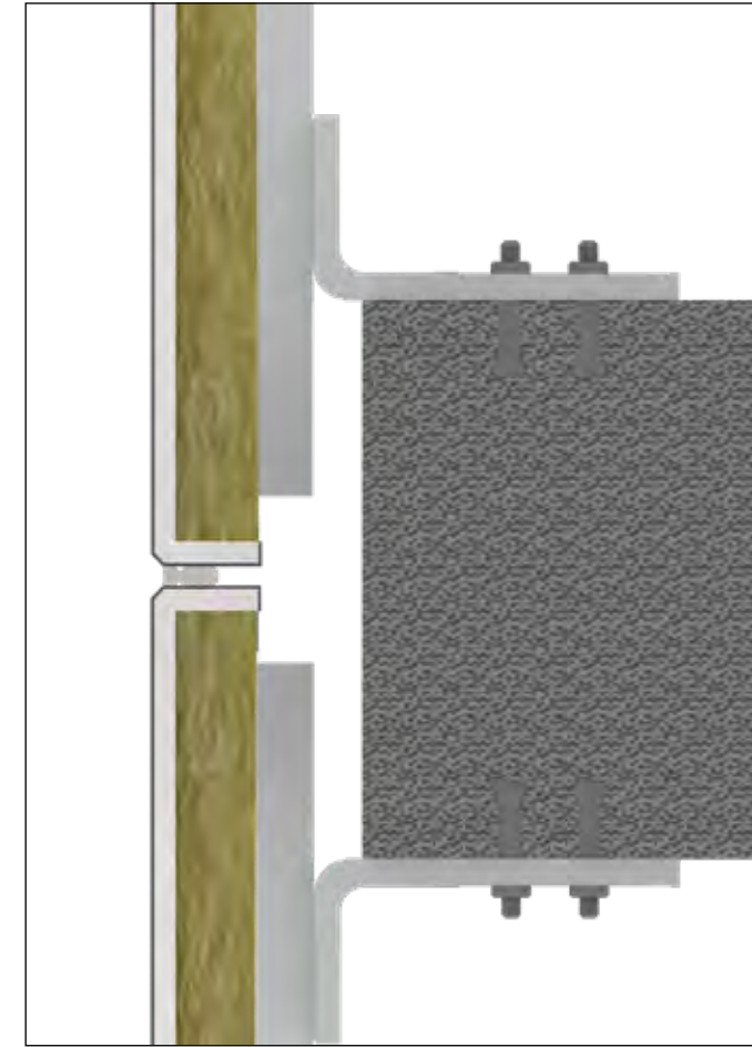
Halfen Bağlantı detayı Halfen fixing detail
