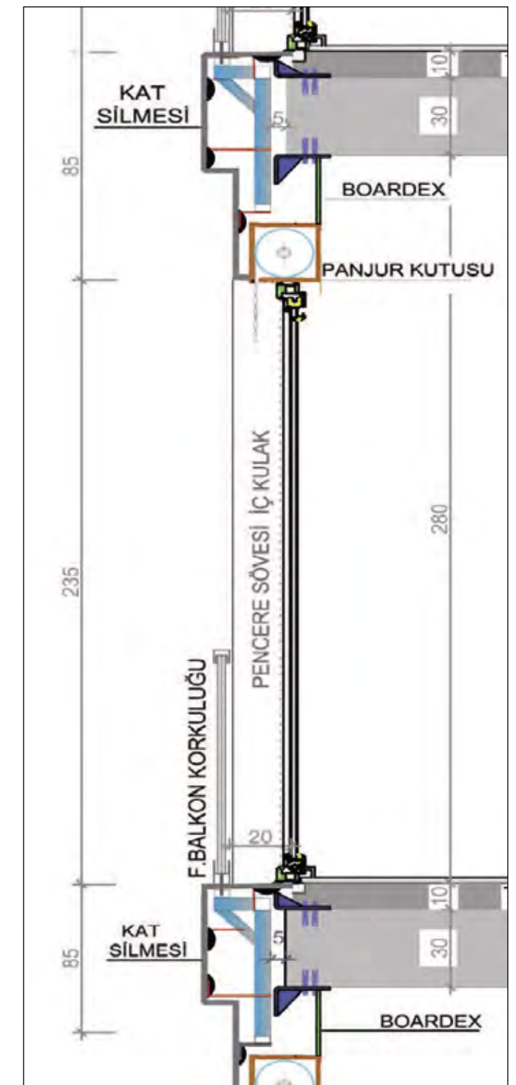
Fransız Balkon Kesiti French Ballcony Section
